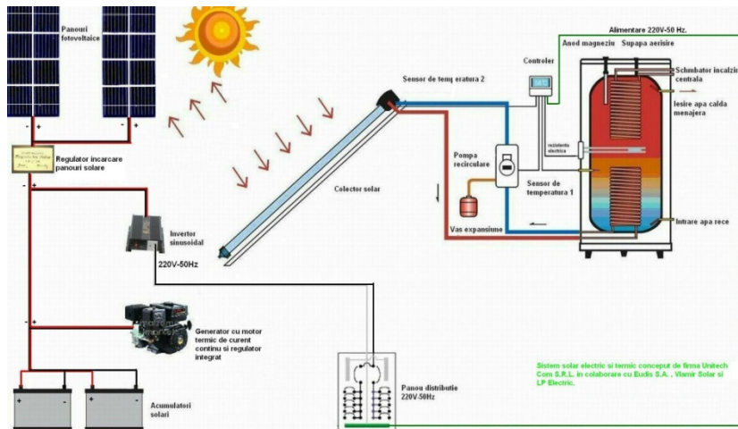
Schema unui panou solar.
